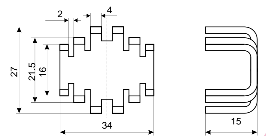
301 27x34x15 mm
