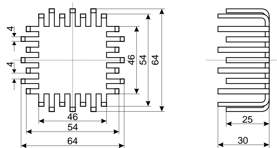
104 64x64x30 mm
