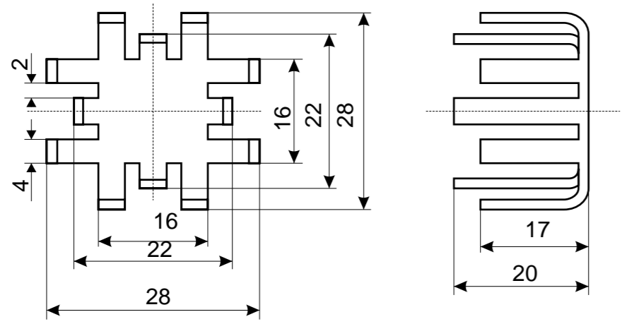
101 28x28x20 mm
