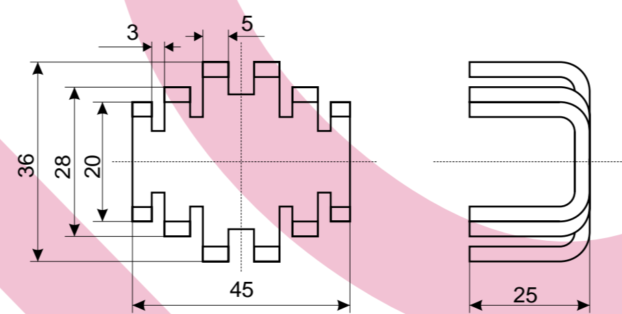
302 36x45x25 mm
